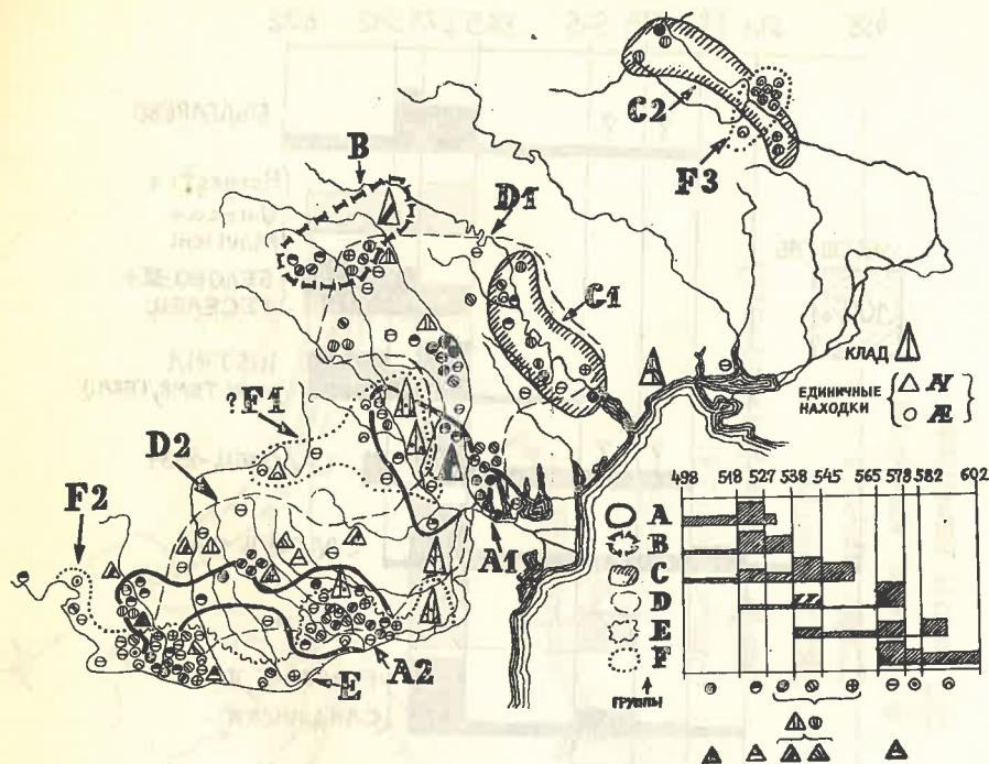
Рис. 1. Корреляция монет
