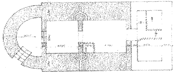
Fig.4. Biserica Adormirii Maicii Domnului. Plan. Nivel subteran. (Foto de arh. S. Ciocanu)
