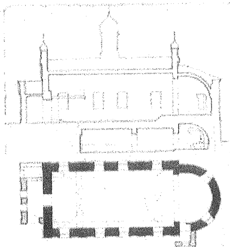
Fig. 5. Biserica Adormirii Maicii Domnului. Plan. Secțiune (de arh. S. Ciocanu)
